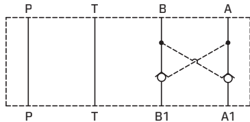
AM5-CP-A
